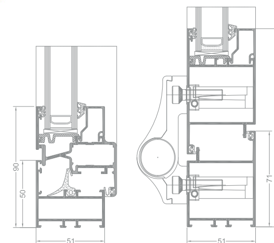
Řez oknem EL 010 + VL 820
