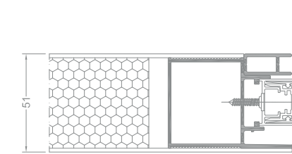
Řez panelovými dveřmi - řešení s padacím prahem
