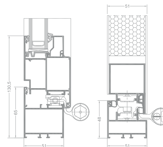
Řez dveřmi EL 011 + EL 022
